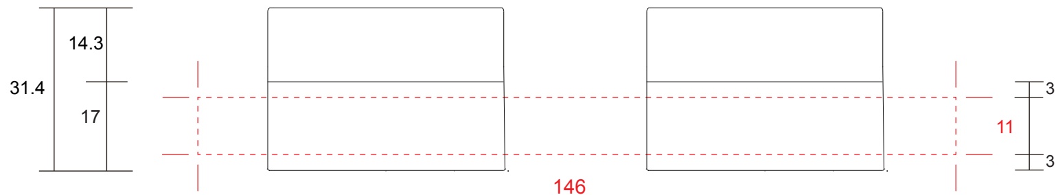
H-20/ Jar Body
